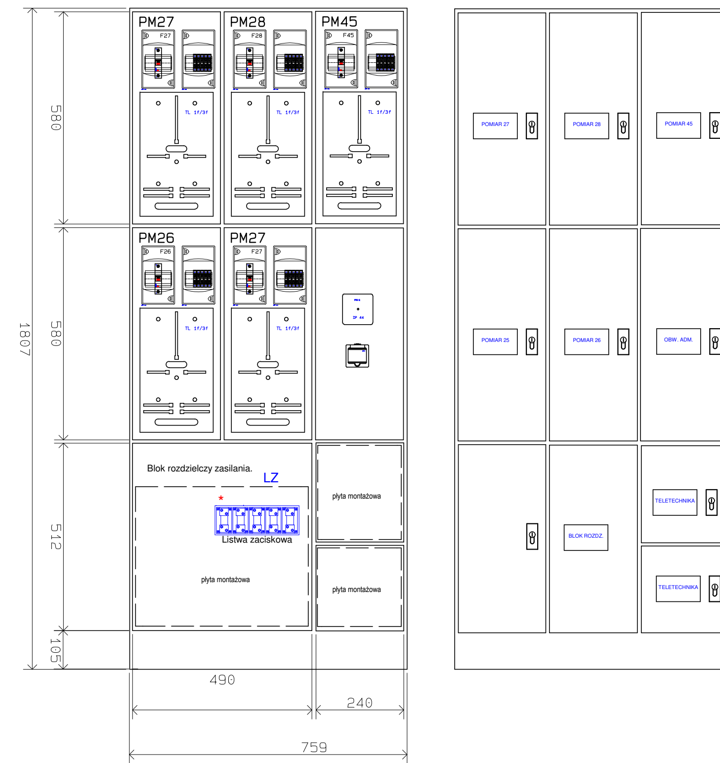
WIDOK MONTAŻOWY ZESTAWU TABLIC POMIAROWYCH ZELP DLA PIĘTRA II KLATKI NR 2 ( DODATKOWY POMIAR )
